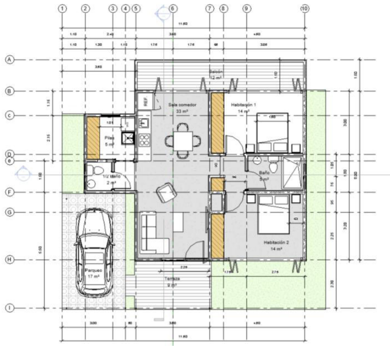
Planta Arquitectónica_Nivel 1
