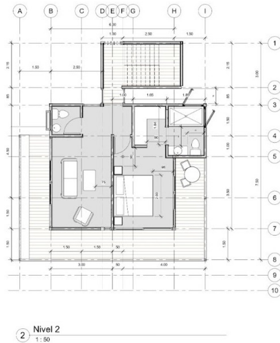
Planta Arquitectónica_Nivel 2
