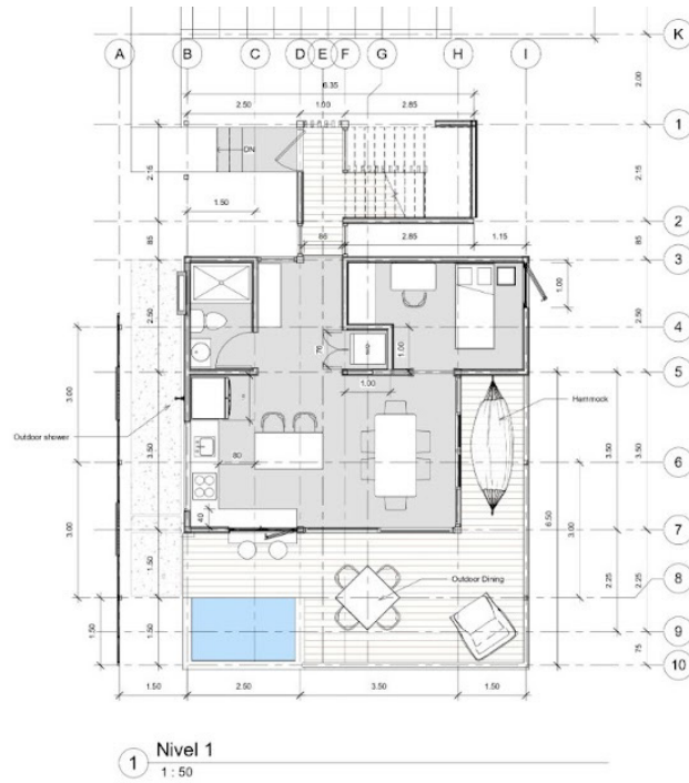
Planta Arquitectónica_Nivel 1
