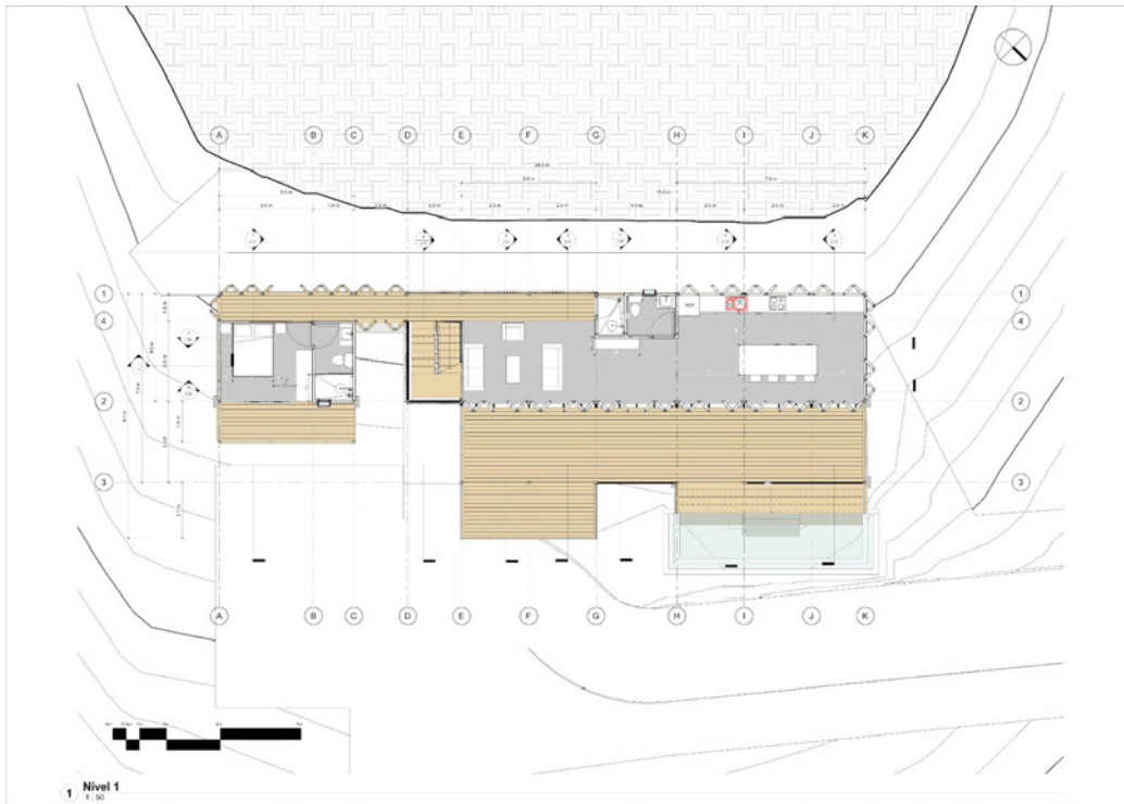
Planta Arquitectónica_Nivel 1
