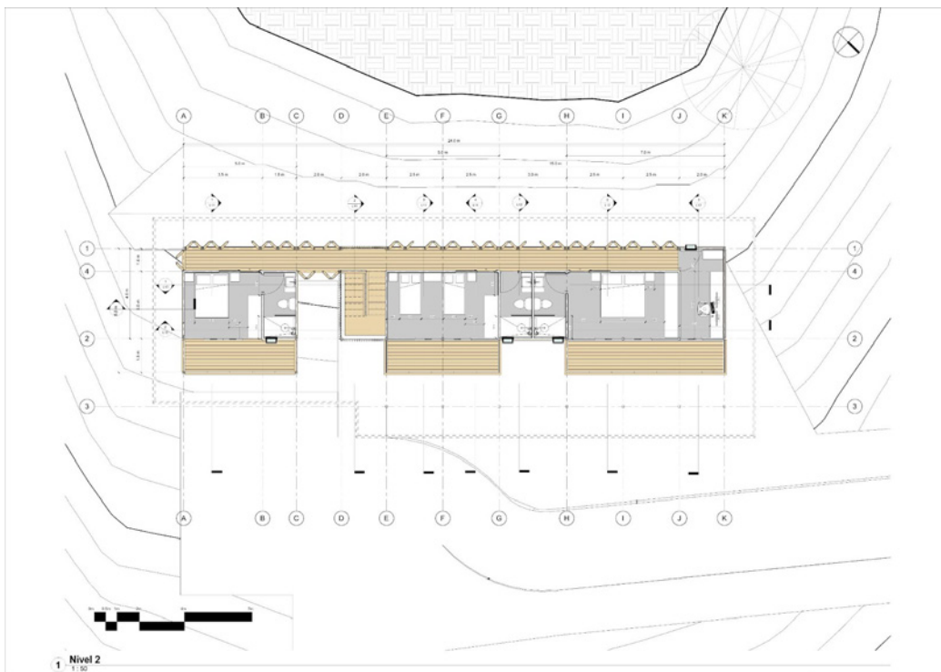
Planta Arquitectónica_Nivel 2
