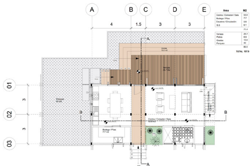
Planta Arquitectónica_Nivel 1
