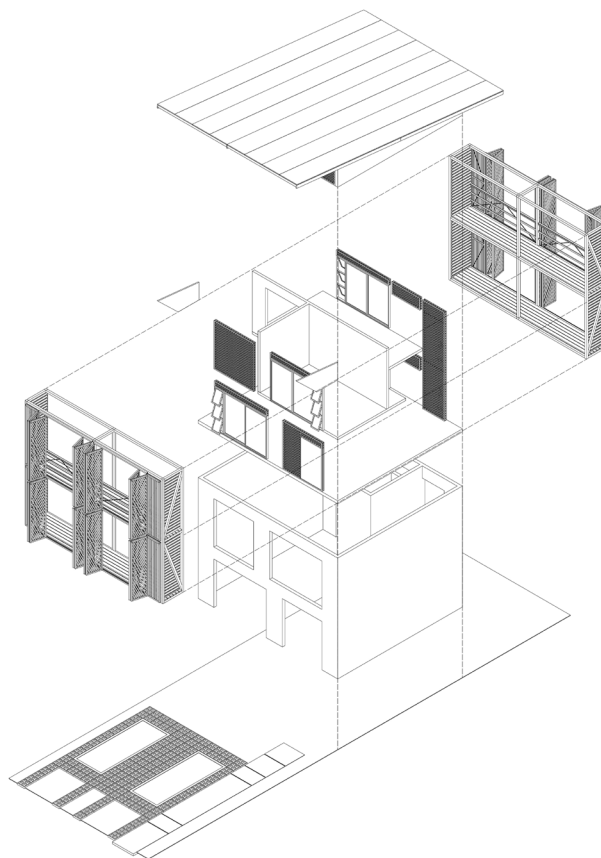
Isométrico
