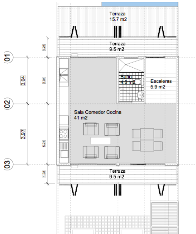
Planta Arquitectónica_Nivel 1
