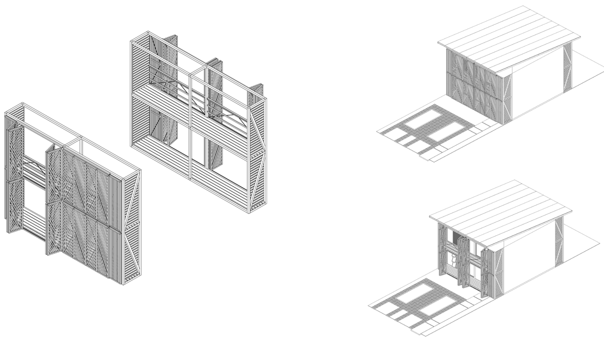
Isométrico
