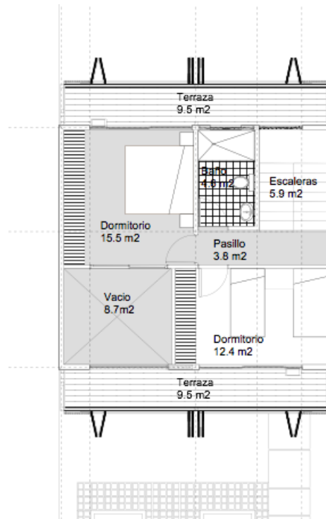
Planta Arquitectónica_Nivel 2
