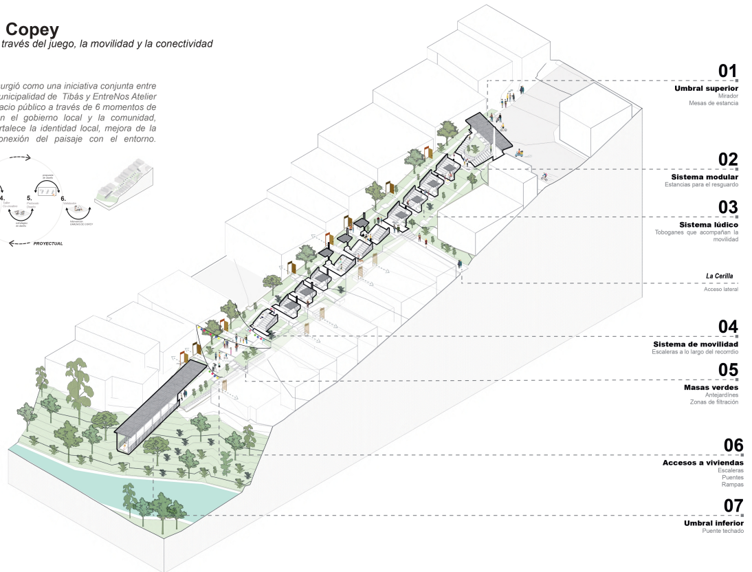
Vista Isométrica
