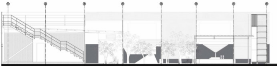
Corte Longitudinal
