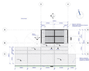
2 A104- N01-Doble 1:50
