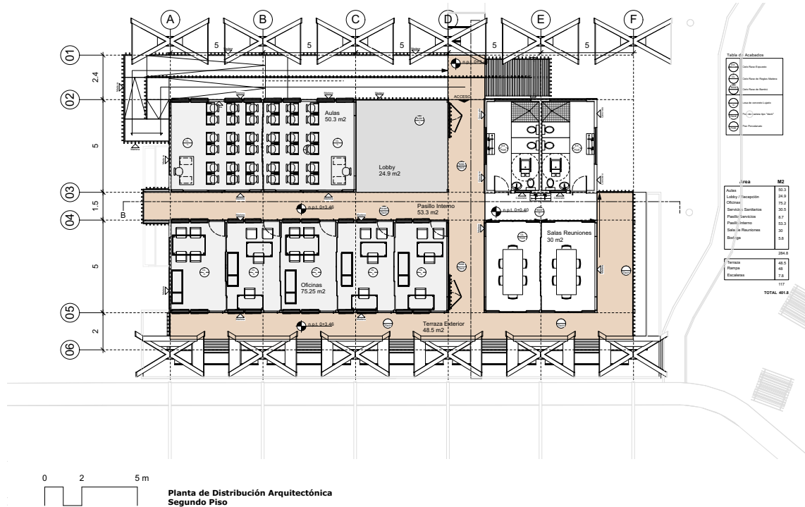
Planta Arquitectónica_Nivel 2
