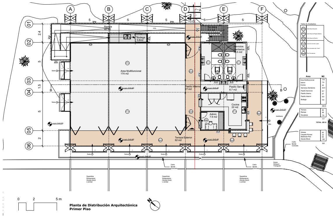
Planta Arquitectónica_Nivel 1
