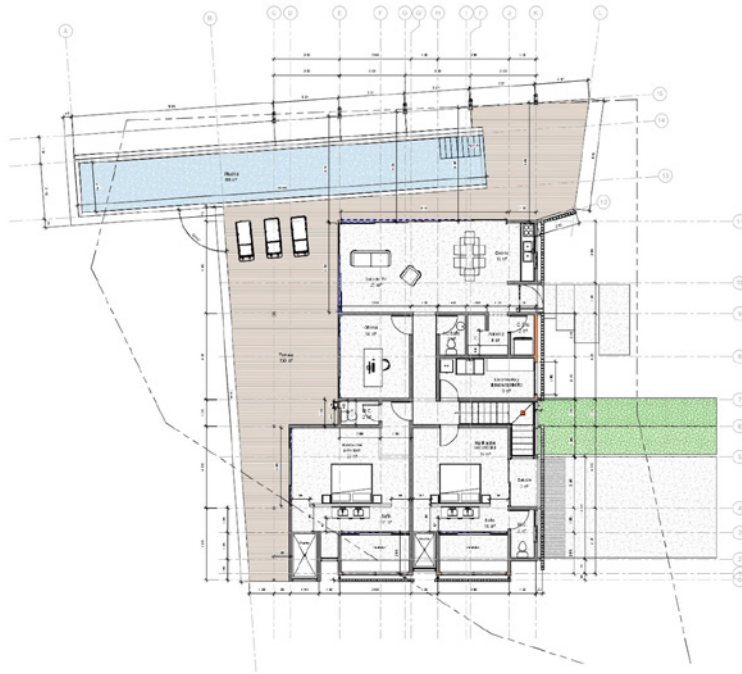
Planta Arquitectónica_Nivel 1
