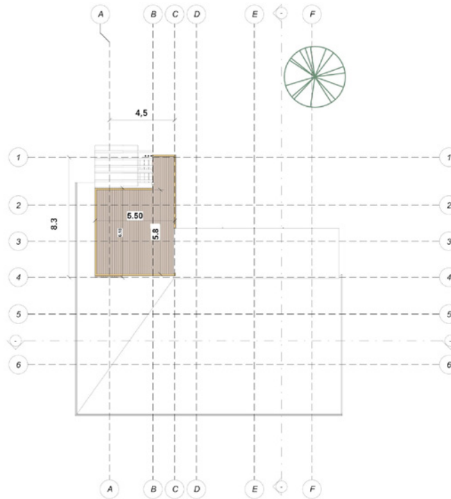
Planta Arquitectónica_Nivel 2
