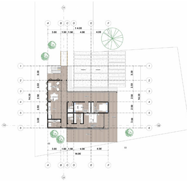
Planta Arquitectónica_Nivel 1
