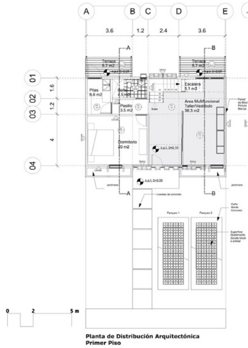
Planta Arquitectónica_Nivel 1
