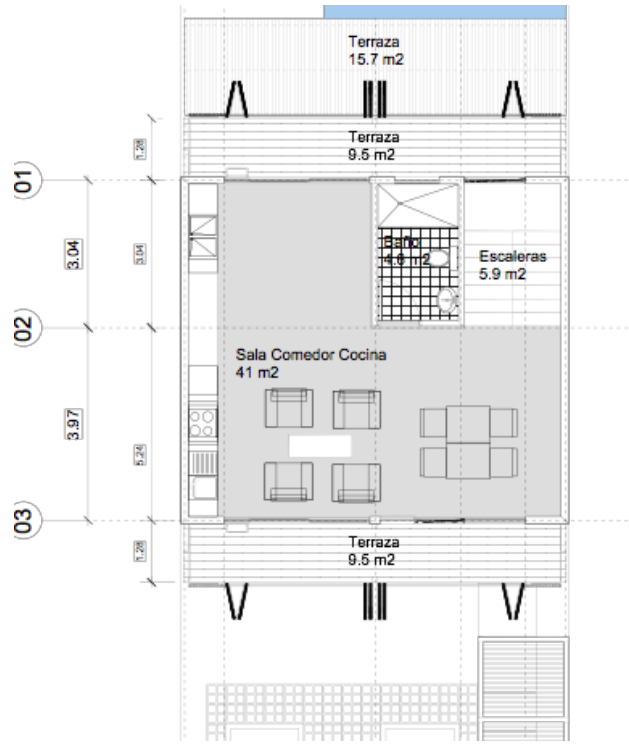
Planta Arquitectónica_Nivel 1
