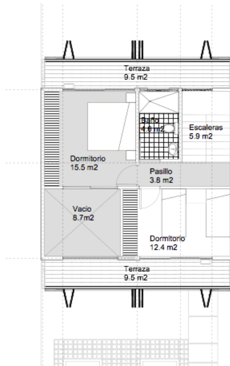
Planta Arquitectónica_Nivel 2
