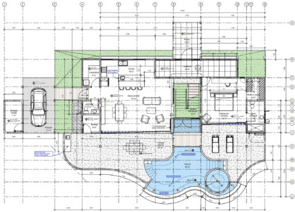
Planta Arquitectónica_Nivel 1
