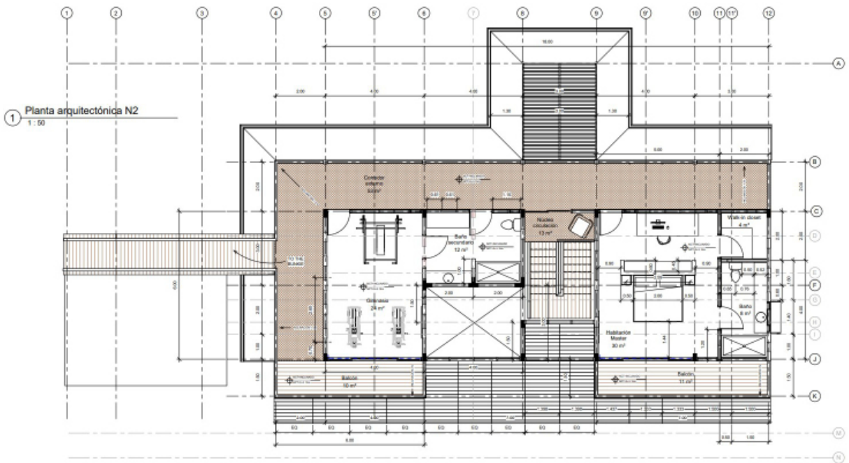
Planta Arquitectónica_Nivel 2
