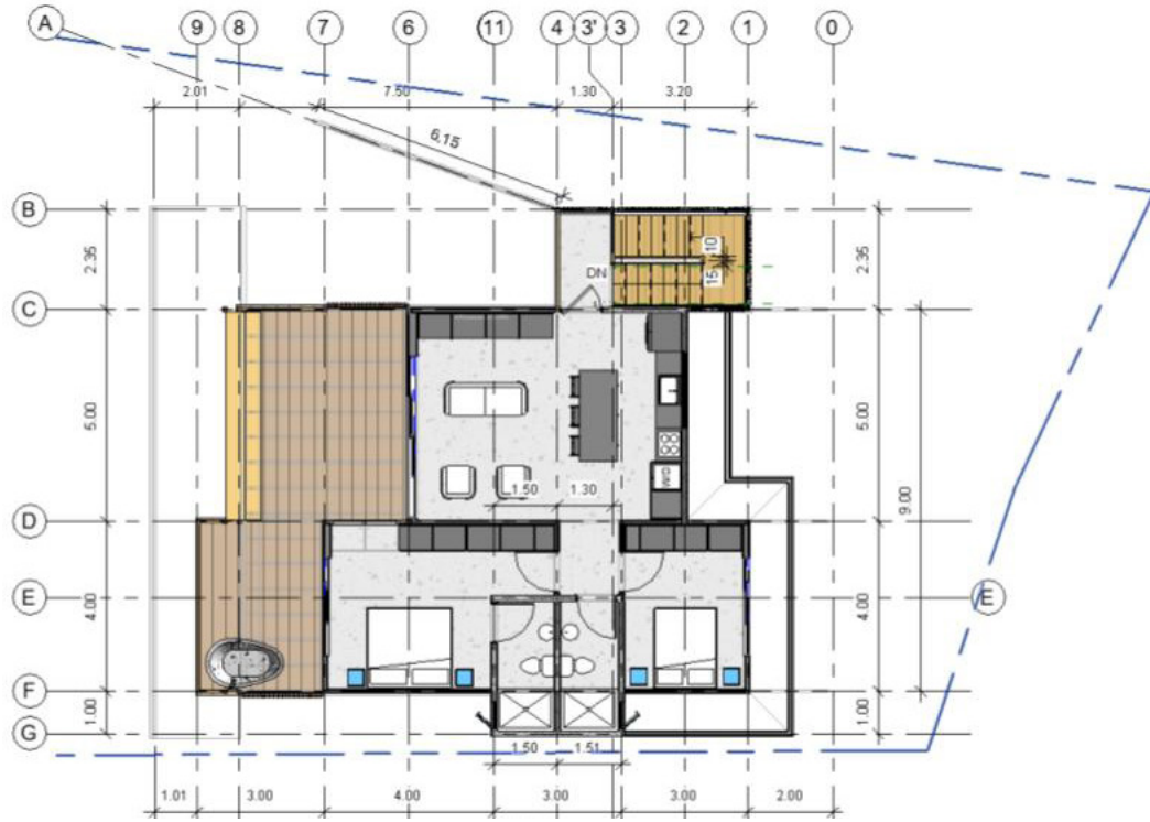
Planta Arquitectónica_Nivel 2
