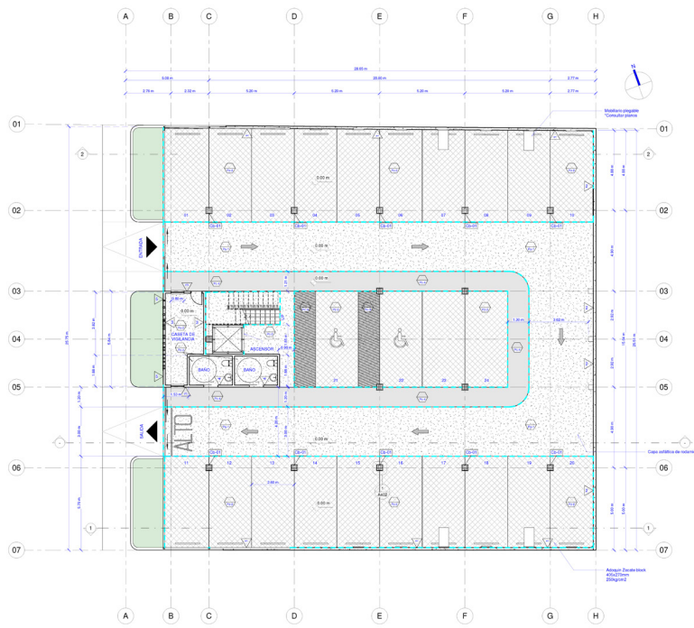
Planta Arquitectónica_Nivel 1
