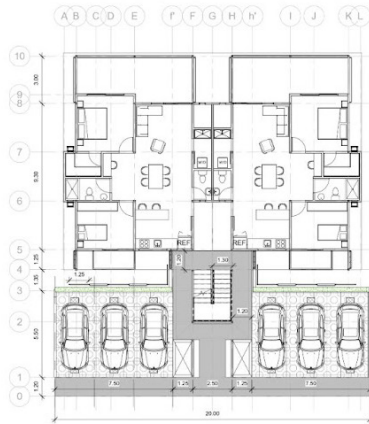
1 NPT 0+0.0m 1:100
