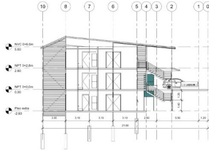
3 Sección transversal 1:100
